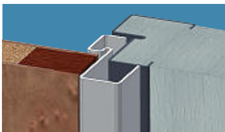
Coupe bloc porte SECURENOV®
